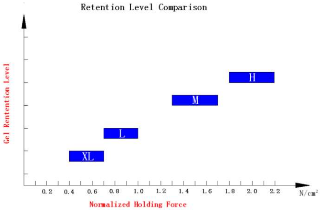
超低粘度、高粘度、中年粘度、低粘度和粘着力曲线图
